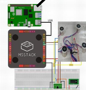
電磁石とその制御
